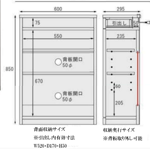
NS-8007 WO/D/WH W600・D295・H850【梱包サイズ:7才】 税込¥53,900 (税抜¥49,000)
