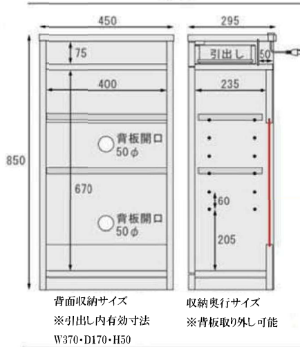
NS-8006 WO/D/WH W450・D295・H850【梱包サイズ:5才】 税込¥49,500 (税抜¥45,000)
