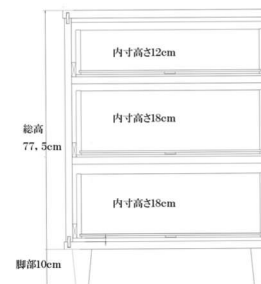
正面内寸図
